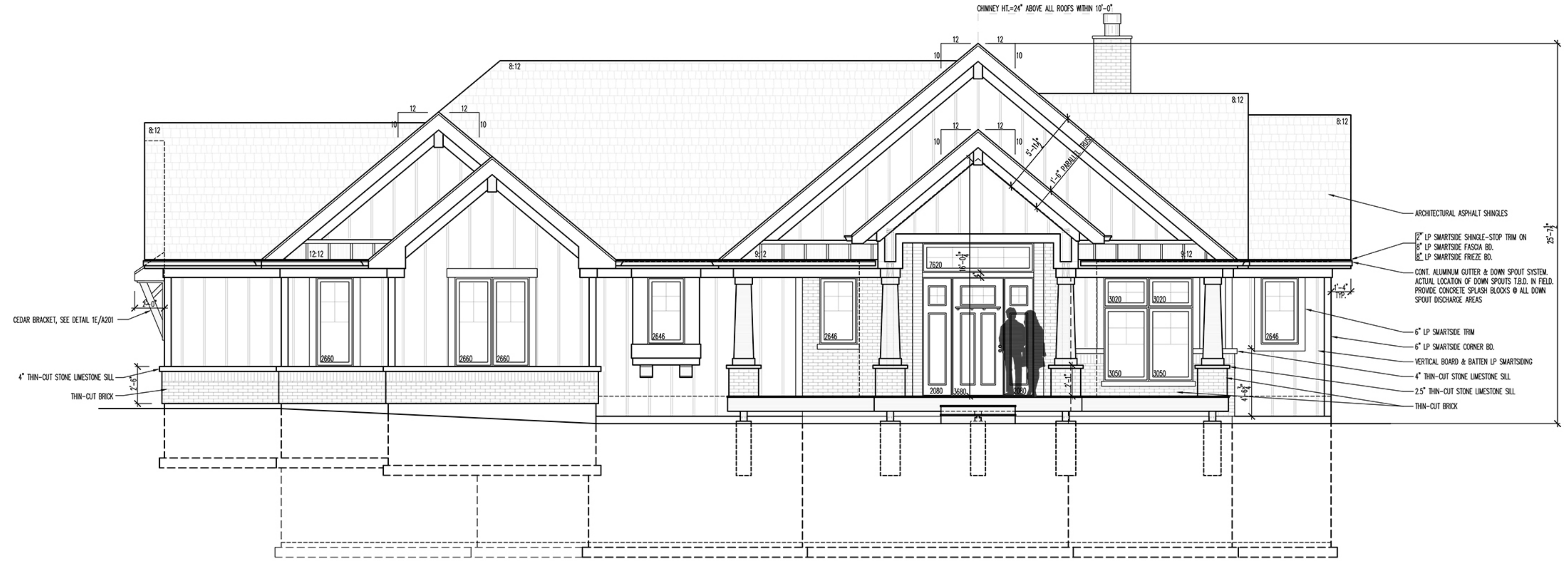
1E A200 FRONT ELEVATION
